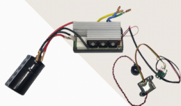
2150-119 PCB (CONTROLLER)
